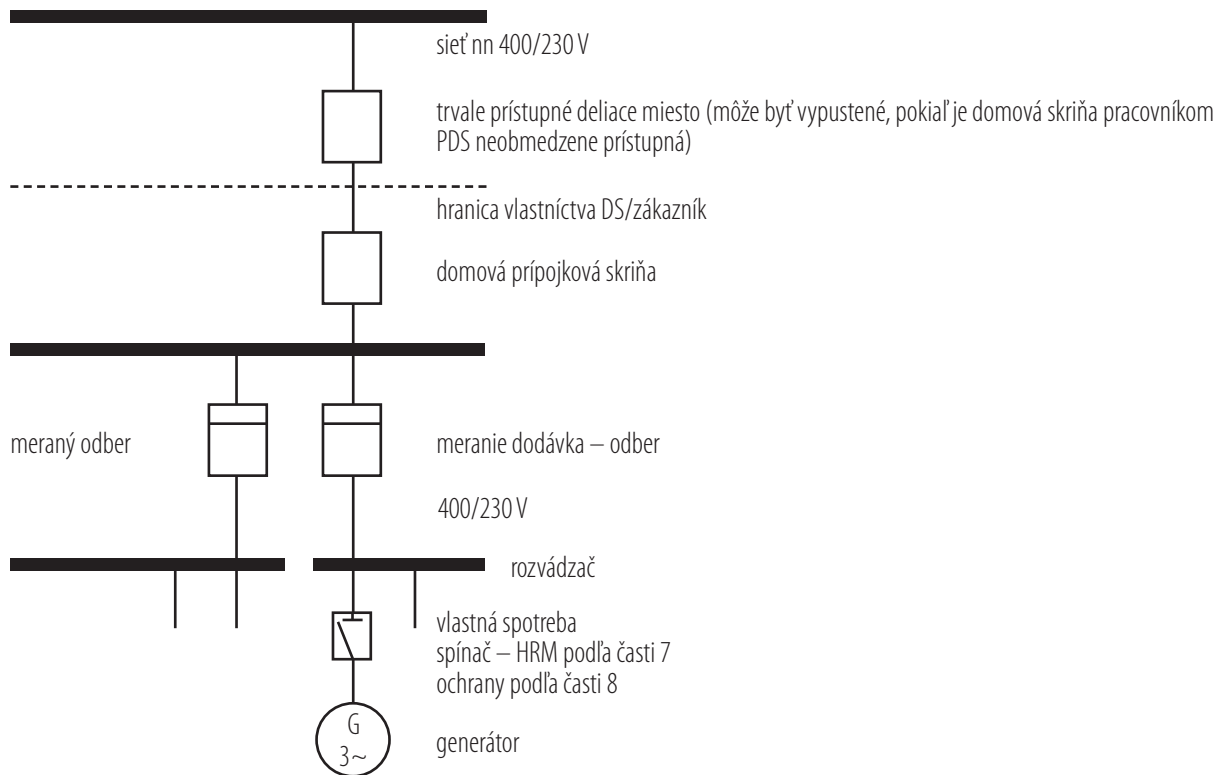
Obrázok 6: Paralelne prevádzkovaná výrobnia v sieti nn bez možnosti ostrovej prevádzky Spoločné pripojenie, možnosť vykázat výrobu a čiastočne ju spotrebovať. Priebehové meranie.
