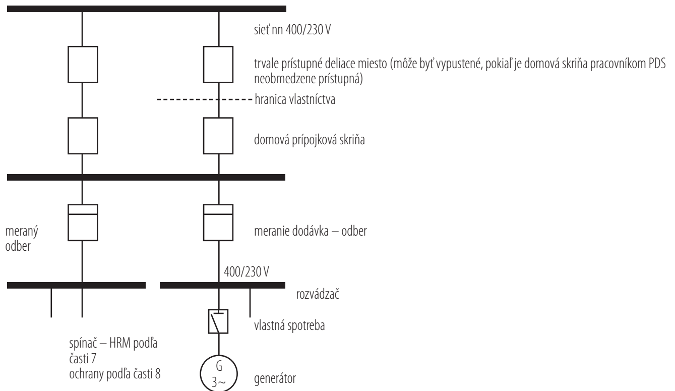
Obrázok 7: Paralelne prevádzkovaná výrobná v sieti nn bez možnosti ostrovnej prevádzky Celá výroba bez vlastnej spotreby dodaná do DS Rozšírenie existujúceho odberu
