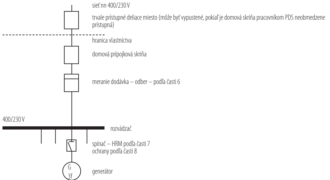
Obrázok 5: Paralelne prevádzkovaná výrobnia v sieti nn bez možnosti ostrovej prevádzky
