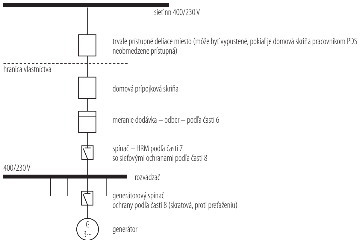
Obrázok 8: Paralelne prevádzkovaná výrobná v sieti nn s možnosťou ostrovej prevádzky
