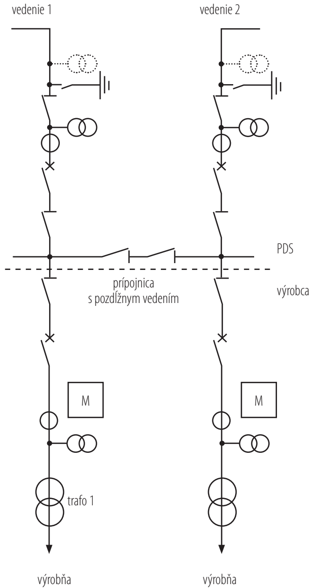
Obr. 13: Pripojenie výroby zaslučkovaním do vedenia 110 kV DS
